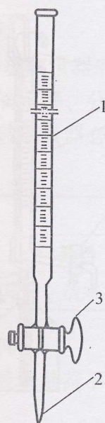
图1 具塞滴定管 1—量管；2—流液口； 3—直通活塞
