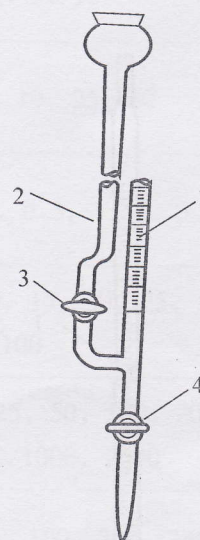
图12 夹式滴定管
